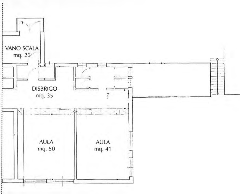
Piano rialzato
